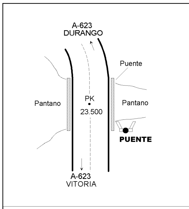
Puente Km. 23,500
