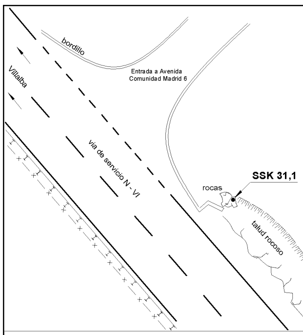
SSK31,1
