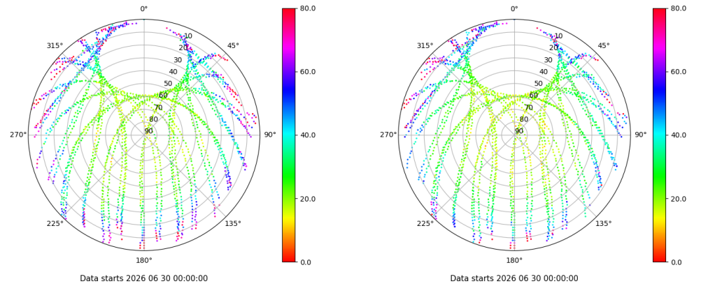
Skyplot for station VIGO. Parameter M1C Data file VIGO00ESP_R_2026181.xtr Skyplot for station VIGO. Parameter M2C Data file VIGO00ESP_R_2026181.xtr
