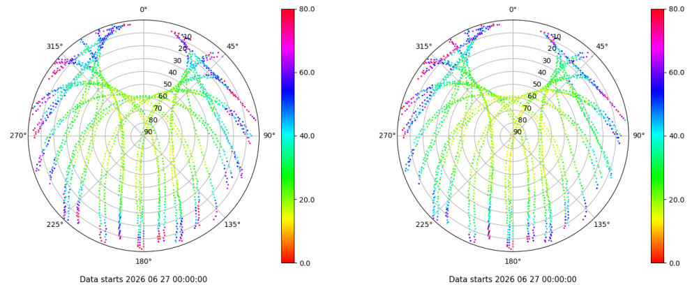
Skyplot for station VIGO. Parameter M1C Data file VIGO00ESP_R_2026178.xtr Skyplot for station VIGO. Parameter M2C Data file VIGO00ESP_R_2026178.xtr
