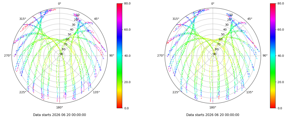
Skyplot for station VIGO. Parameter M1C Data file VIGO00ESP_R_2026171.xtr Skyplot for station VIGO. Parameter M2C Data file VIGO00ESP_R_2026171.xtr
