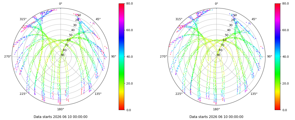
Skyplot for station VIGO. Parameter M1C Data file VIGO00ESP_R_2026161.xtr Skyplot for station VIGO. Parameter M2C Data file VIGO00ESP_R_2026161.xtr
