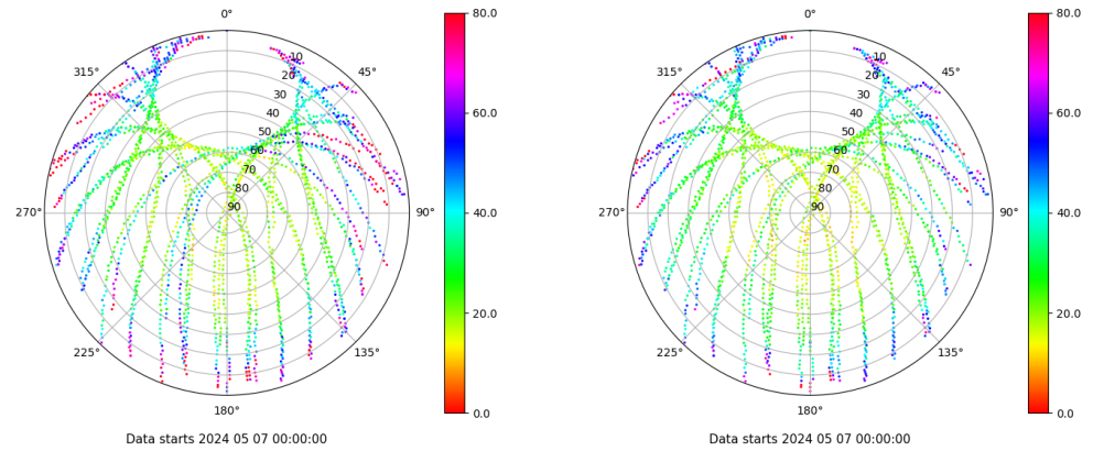
Skyplot for station VIGO. Parameter M1C Data file VIGO00ESP_R_2024128.xtr Skyplot for station VIGO. Parameter M2C Data file VIGO00ESP_R_2024128.xtr
