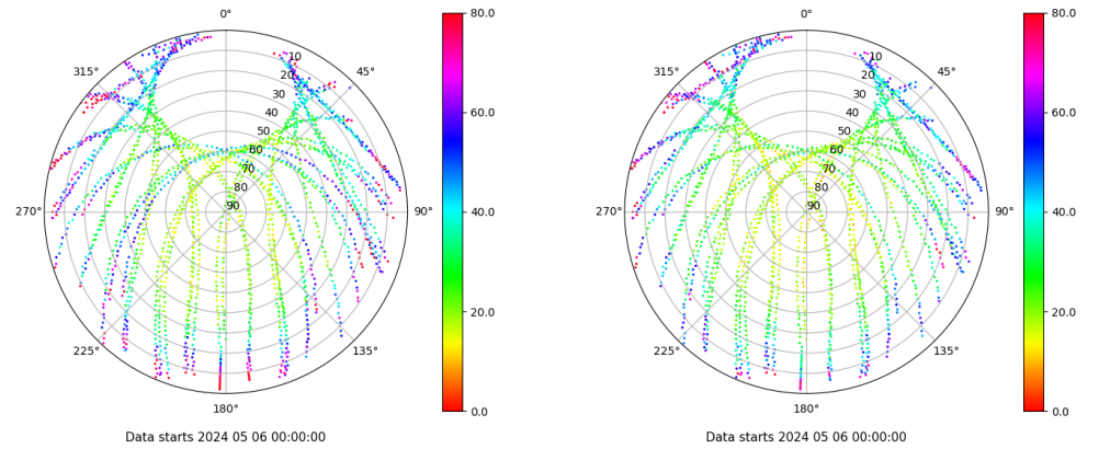
Skyplot for station VIGO. Parameter M1C Data file VIGO00ESP_R_2024127.xtr Skyplot for station VIGO. Parameter M2C Data file VIGO00ESP_R_2024127.xtr
