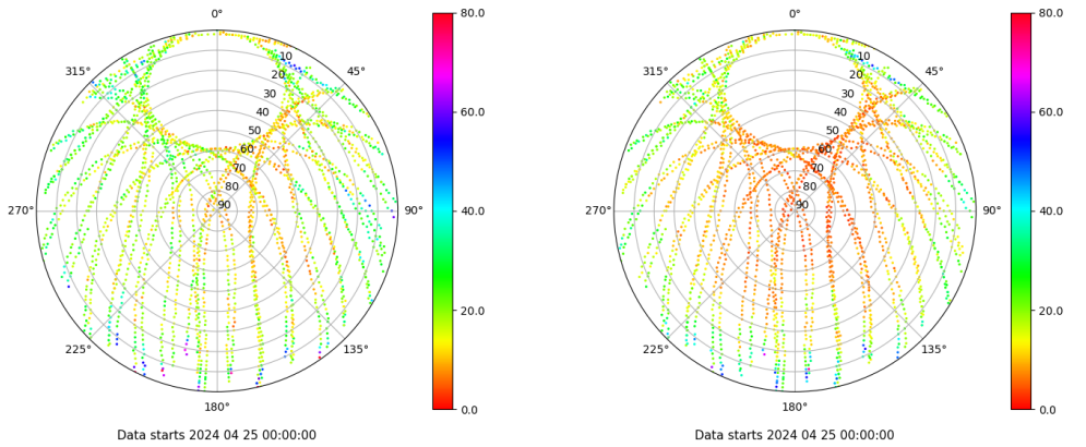
Skyplot for station VALA. Parameter M1C Data file VALA00ESP_R_2024116.xtr Skyplot for station VALA. Parameter M2C Data file VALA00ESP_R_2024116.xtr
