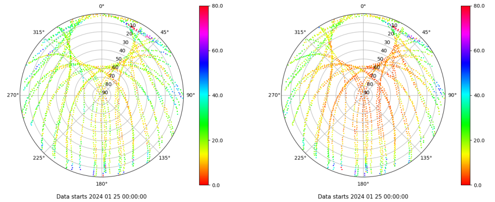
Skyplot for station VALA. Parameter M1C Data file VALA00ESP_R_2024025.xtr Skyplot for station VALA. Parameter M2C Data file VALA00ESP_R_2024025.xtr
