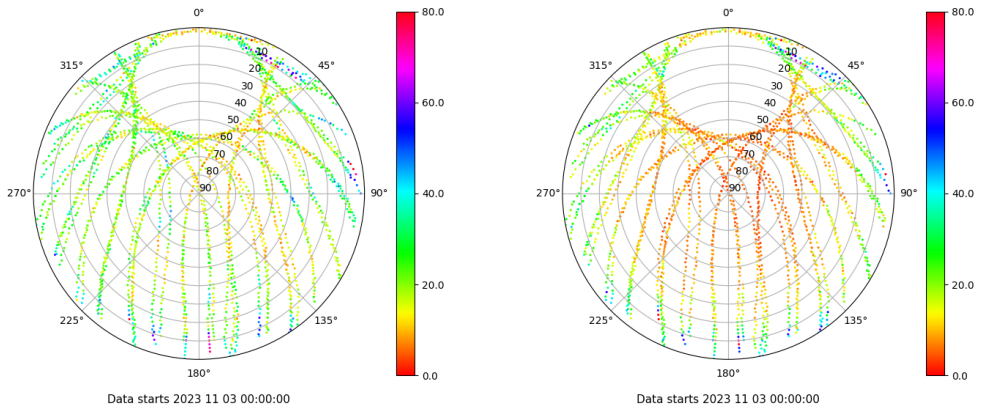
Skyplot for station VALA. Parameter M1C Data file VALA00ESP_R_2023307.xtr Skyplot for station VALA. Parameter M2C Data file VALA00ESP_R_2023307.xtr
