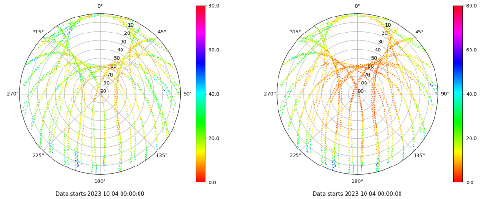
Skyplot for station VALA. Parameter M1C Data file VALA00ESP_R_2023277.xtr Skyplot for station VALA. Parameter M2C Data file VALA00ESP_R_2023277.xtr
