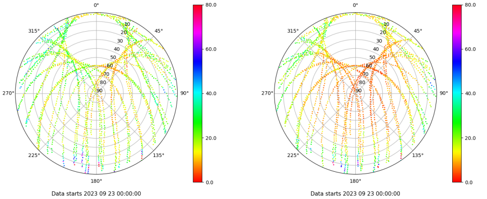
Skyplot for station VALA. Parameter M1C Data file VALA00ESP_R_2023266.xtr Skyplot for station VALA. Parameter M2C Data file VALA00ESP_R_2023266.xtr
