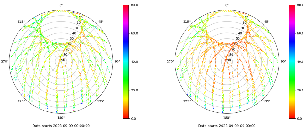
Skyplot for station VALA. Parameter M1C Data file VALA00ESP_R_2023252.xtr Skyplot for station VALA. Parameter M2C Data file VALA00ESP_R_2023252.xtr
