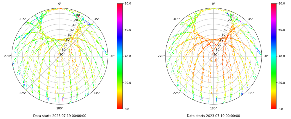
Skyplot for station VALA. Parameter M1C Data file VALA00ESP_R_2023200.xtr Skyplot for station VALA. Parameter M2C Data file VALA00ESP_R_2023200.xtr
