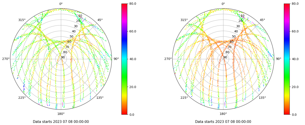
Skyplot for station VALA. Parameter M1C Data file VALA00ESP_R_2023189.xtr Skyplot for station VALA. Parameter M2C Data file VALA00ESP_R_2023189.xtr
