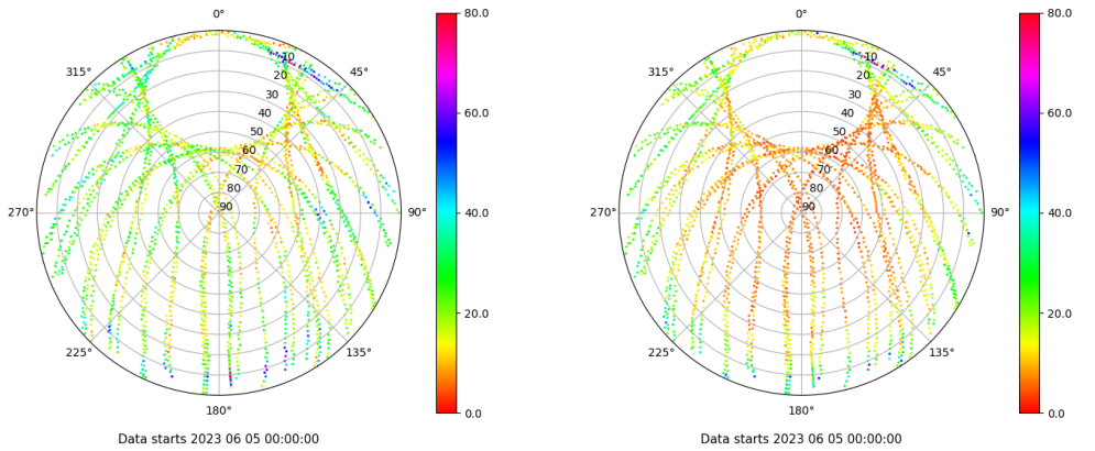
Skyplot for station VALA. Parameter M1C Data file VALA00ESP_R_2023156.xtr Skyplot for station VALA. Parameter M2C Data file VALA00ESP_R_2023156.xtr
