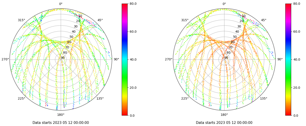
Skyplot for station VALA. Parameter M1C Data file VALA00ESP_R_2023132.xtr Skyplot for station VALA. Parameter M2C Data file VALA00ESP_R_2023132.xtr
