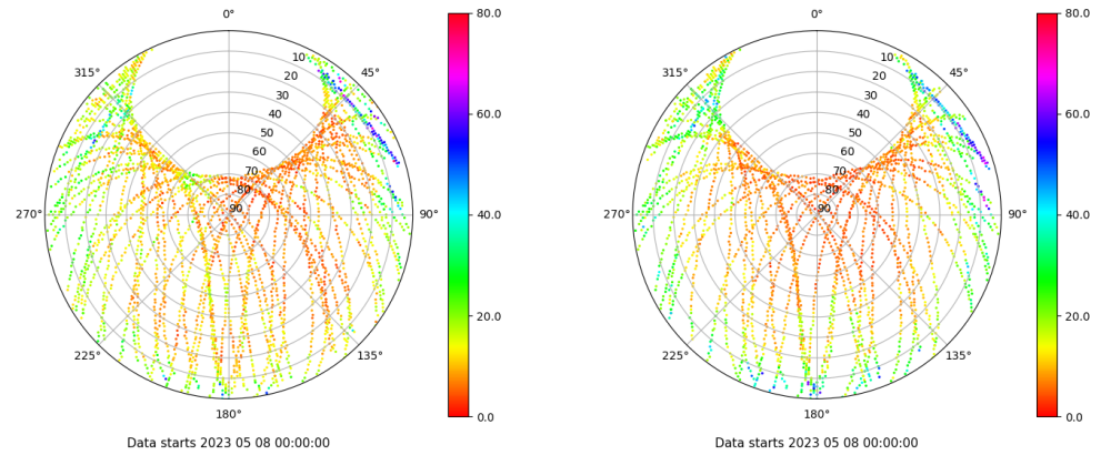
Skyplot for station VALA. Parameter M1C Data file VALA00ESP_R_2023128.xtr Skyplot for station VALA. Parameter M2S Data file VALA00ESP_R_2023128.xtr
