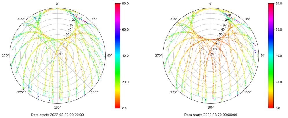
Skyplot for station VALA. Parameter M1C Data file VALA00ESP_R_2022232.xtr Skyplot for station VALA. Parameter M2C Data file VALA00ESP_R_2022232.xtr
