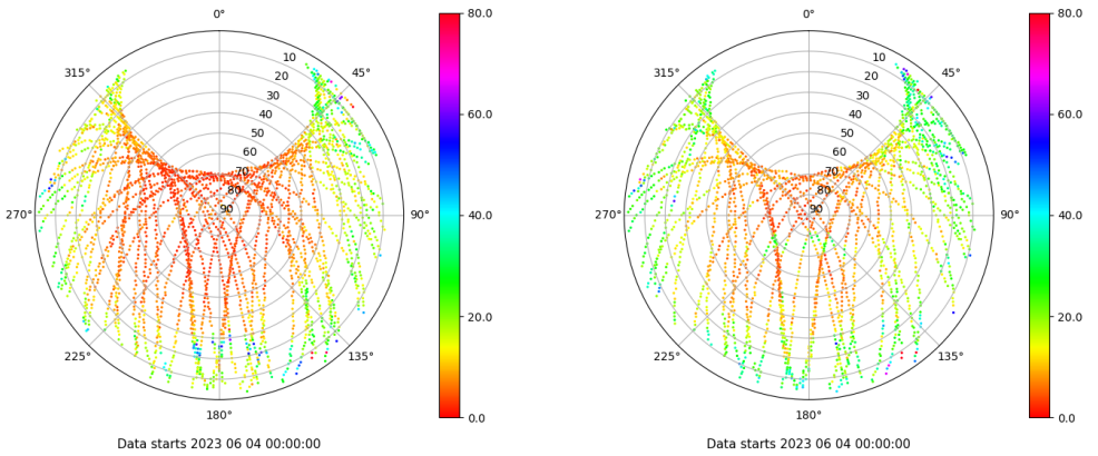
Skyplot for station TERU. Parameter M1C Data file TERU00ESP_R_2023155.xtr Skyplot for station TERU. Parameter M2S Data file TERU00ESP_R_2023155.xtr
