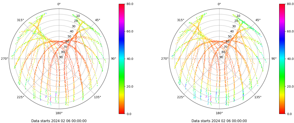
Skyplot for station TARR. Parameter M1C Data file TARR00ESP_R_2024037.xtr Skyplot for station TARR. Parameter M2P Data file TARR00ESP_R_2024037.xtr
