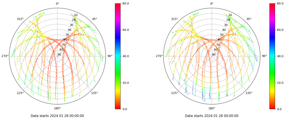
Skyplot for station TARR. Parameter M1C Data file TARR00ESP_R_2024028.xtr Skyplot for station TARR. Parameter M2P Data file TARR00ESP_R_2024028.xtr
