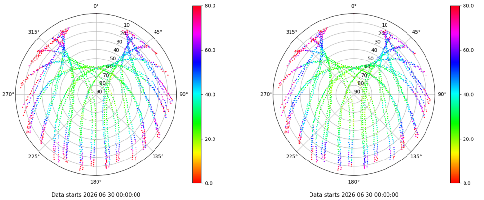
Skyplot for station PUIG. Parameter M1C Data file PUIG00ESP_R_2026181.xtr Skyplot for station PUIG. Parameter M2C Data file PUIG00ESP_R_2026181.xtr
