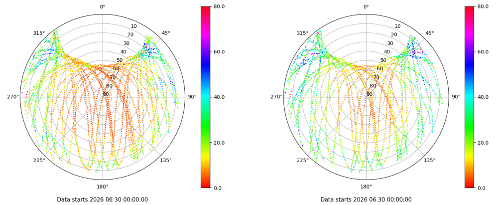
Skyplot for station LPAL. Parameter M1C Data file LPAL00ESP_R_2026181.xtr Skyplot for station LPAL. Parameter M2S Data file LPAL00ESP_R_2026181.xtr
