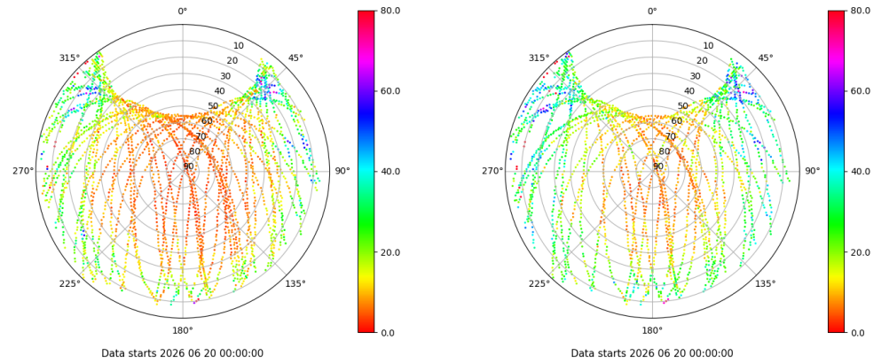
Skyplot for station LPAL. Parameter M1C Data file LPAL00ESP_R_2026171.xtr Skyplot for station LPAL. Parameter M2S Data file LPAL00ESP_R_2026171.xtr
