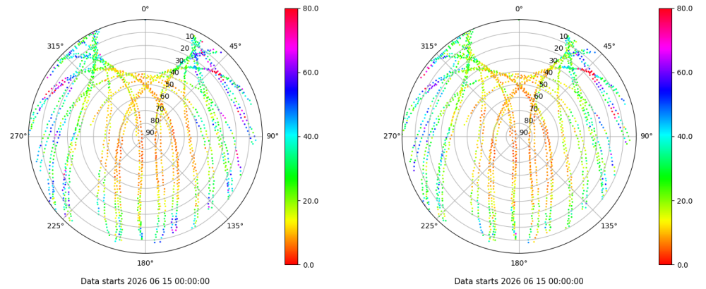
Skyplot for station LPAL. Parameter M1C Data file LPAL00ESP_R_2026166.xtr Skyplot for station LPAL. Parameter M2C Data file LPAL00ESP_R_2026166.xtr
