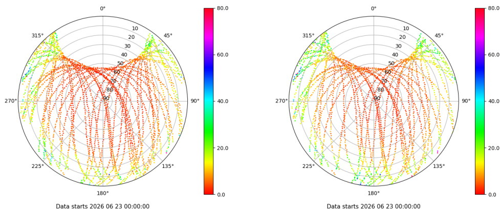
Skyplot for station IZAN. Parameter M1C Data file IZAN00ESP_R_2026174.xtr Skyplot for station IZAN. Parameter M2S Data file IZAN00ESP_R_2026174.xtr
