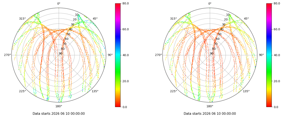
Skyplot for station IZAN. Parameter M1C Data file IZAN00ESP_R_2026161.xtr Skyplot for station IZAN. Parameter M2C Data file IZAN00ESP_R_2026161.xtr
