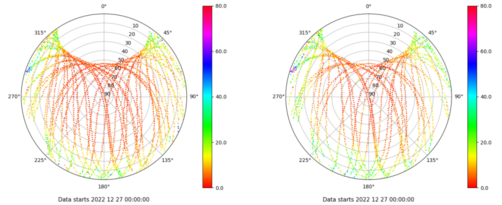
Skyplot for station IZAN. Parameter M1C Data file IZAN00ESP_R_2022361.xtr Skyplot for station IZAN. Parameter M2S Data file IZAN00ESP_R_2022361.xtr
