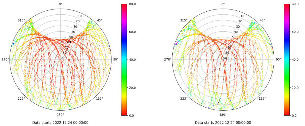
Skyplot for station IZAN. Parameter M1C Data file IZAN00ESP_R_2022358.xtr Skyplot for station IZAN. Parameter M2S Data file IZAN00ESP_R_2022358.xtr
