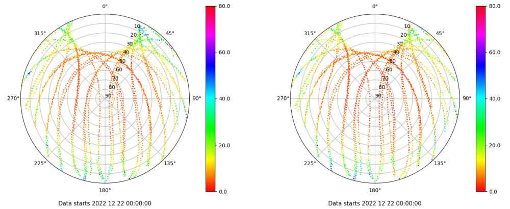
Skyplot for station IZAN. Parameter M1C Data file IZAN00ESP_R_2022356.xtr Skyplot for station IZAN. Parameter M2C Data file IZAN00ESP_R_2022356.xtr
