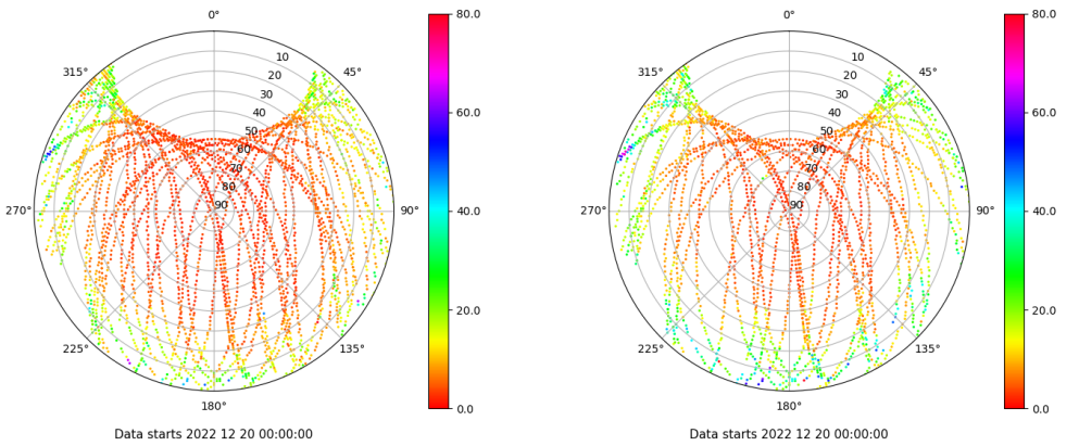
Skyplot for station IZAN. Parameter M1C Data file IZAN00ESP_R_2022354.xtr Skyplot for station IZAN. Parameter M2S Data file IZAN00ESP_R_2022354.xtr
