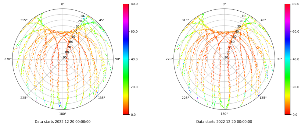
Skyplot for station IZAN. Parameter M1C Data file IZAN00ESP_R_2022354.xtr Skyplot for station IZAN. Parameter M2C Data file IZAN00ESP_R_2022354.xtr
