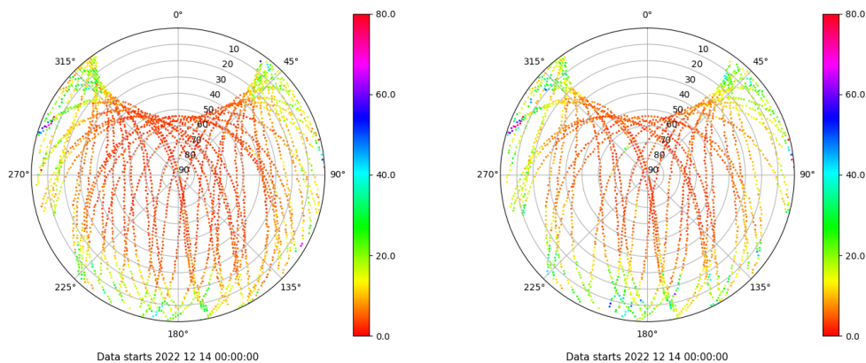
Skyplot for station IZAN. Parameter M1C Data file IZAN00ESP_R_2022348.xtr Skyplot for station IZAN. Parameter M2S Data file IZAN00ESP_R_2022348.xtr
