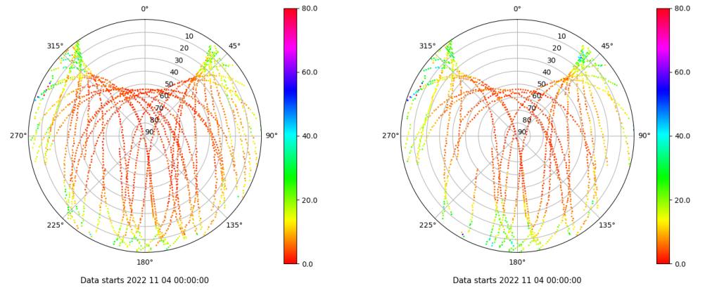
Skyplot for station IZAN. Parameter M1C Data file IZAN00ESP_R_2022308.xtr Skyplot for station IZAN. Parameter M2S Data file IZAN00ESP_R_2022308.xtr
