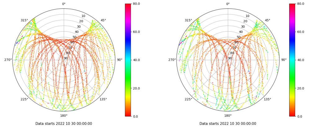
Skyplot for station IZAN. Parameter M1C Data file IZAN00ESP_R_2022303.xtr Skyplot for station IZAN. Parameter M2S Data file IZAN00ESP_R_2022303.xtr
