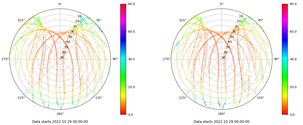
Skyplot for station IZAN. Parameter M1C Data file IZAN00ESP_R_2022302.xtr Skyplot for station IZAN. Parameter M2C Data file IZAN00ESP_R_2022302.xtr
