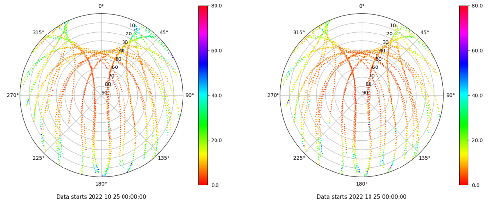
Skyplot for station IZAN. Parameter M1C Data file IZAN00ESP_R_2022298.xtr Skyplot for station IZAN. Parameter M2C Data file IZAN00ESP_R_2022298.xtr
