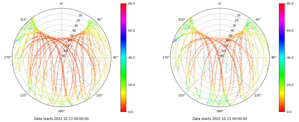
Skyplot for station IZAN. Parameter M1C Data file IZAN00ESP_R_2022296.xtr Skyplot for station IZAN. Parameter M2S Data file IZAN00ESP_R_2022296.xtr
