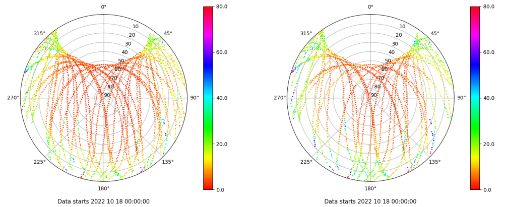
Skyplot for station IZAN. Parameter M1C Data file IZAN00ESP_R_2022291.xtr Skyplot for station IZAN. Parameter M2S Data file IZAN00ESP_R_2022291.xtr
