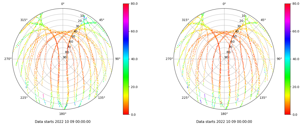
Skyplot for station IZAN. Parameter M1C Data file IZAN00ESP_R_2022282.xtr Skyplot for station IZAN. Parameter M2C Data file IZAN00ESP_R_2022282.xtr
