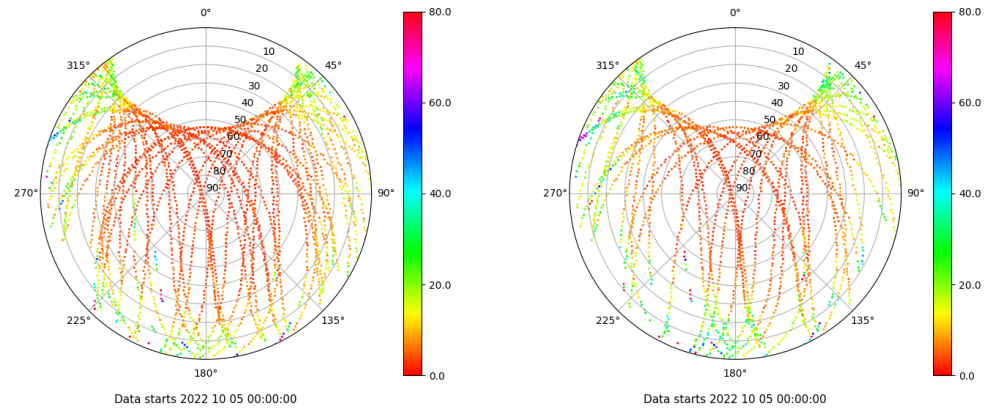
Skyplot for station IZAN. Parameter M1C Data file IZAN00ESP_R_2022278.xtr Skyplot for station IZAN. Parameter M2S Data file IZAN00ESP_R_2022278.xtr
