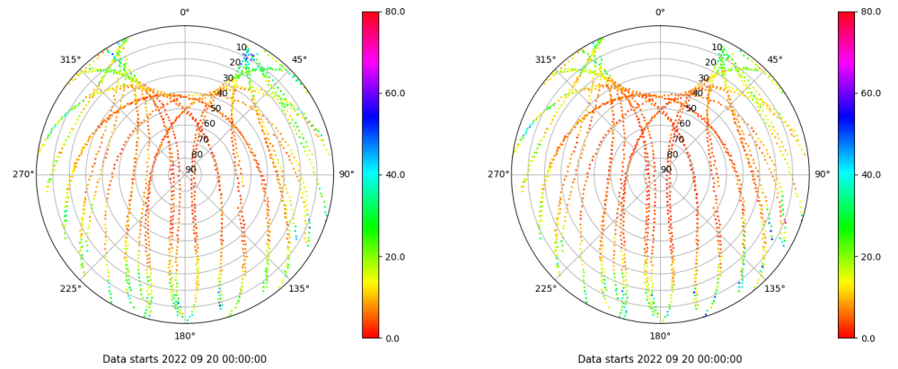
Skyplot for station IZAN. Parameter M1C Data file IZAN00ESP_R_2022263.xtr Skyplot for station IZAN. Parameter M2C Data file IZAN00ESP_R_2022263.xtr
