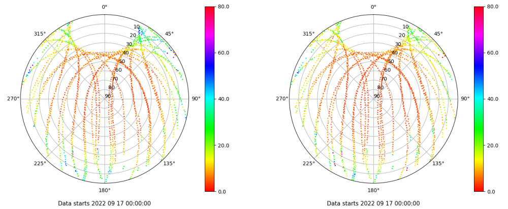
Skyplot for station IZAN. Parameter M1C Data file IZAN00ESP_R_2022260.xtr Skyplot for station IZAN. Parameter M2C Data file IZAN00ESP_R_2022260.xtr
