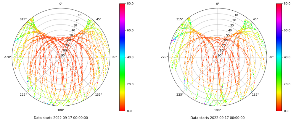
Skyplot for station IZAN. Parameter M1C Data file IZAN00ESP_R_2022260.xtr Skyplot for station IZAN. Parameter M2S Data file IZAN00ESP_R_2022260.xtr
