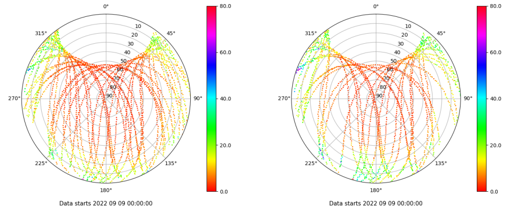
Skyplot for station IZAN. Parameter M1C Data file IZAN00ESP_R_2022252.xtr Skyplot for station IZAN. Parameter M2S Data file IZAN00ESP_R_2022252.xtr
