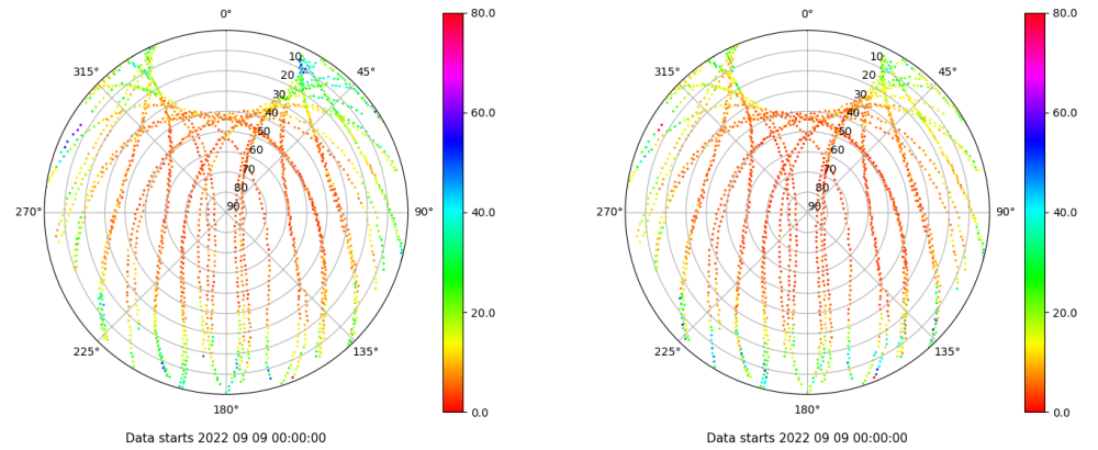
Skyplot for station IZAN. Parameter M1C Data file IZAN00ESP_R_2022252.xtr Skyplot for station IZAN. Parameter M2C Data file IZAN00ESP_R_2022252.xtr
