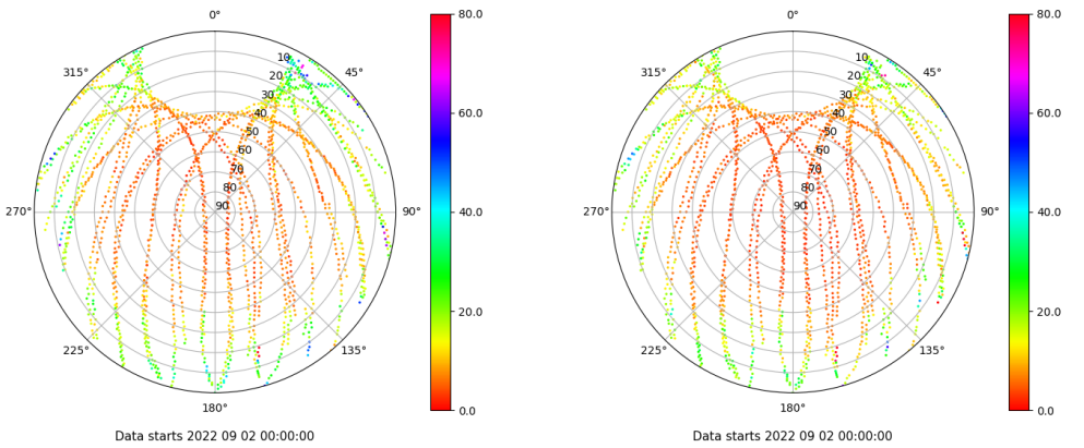
Skyplot for station IZAN. Parameter M1C Data file IZAN00ESP_R_2022245.xtr Skyplot for station IZAN. Parameter M2C Data file IZAN00ESP_R_2022245.xtr
