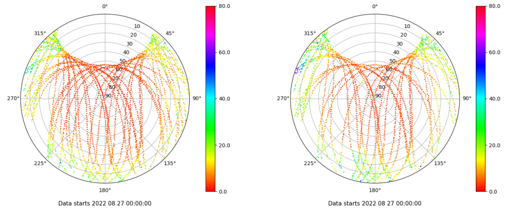
Skyplot for station IZAN. Parameter M1C Data file IZAN00ESP_R_2022239.xtr Skyplot for station IZAN. Parameter M2S Data file IZAN00ESP_R_2022239.xtr
