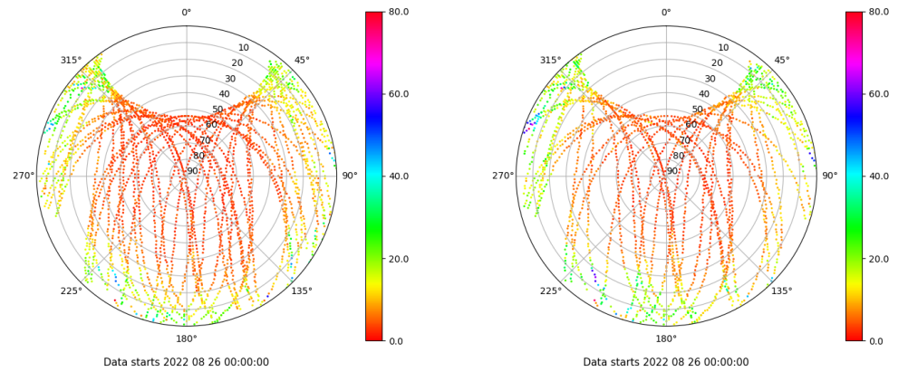
Skyplot for station IZAN. Parameter M1C Data file IZAN00ESP_R_2022238.xtr Skyplot for station IZAN. Parameter M2S Data file IZAN00ESP_R_2022238.xtr
