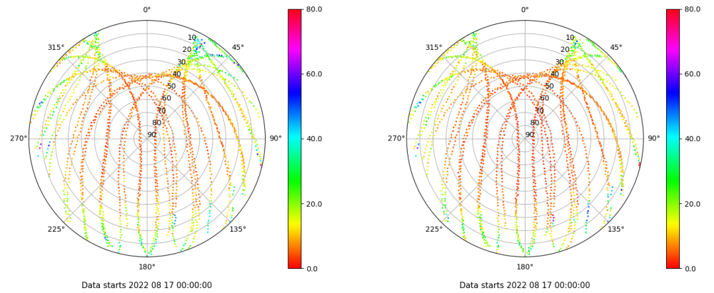
Skyplot for station IZAN. Parameter M1C Data file IZAN00ESP_R_2022229.xtr Skyplot for station IZAN. Parameter M2C Data file IZAN00ESP_R_2022229.xtr
