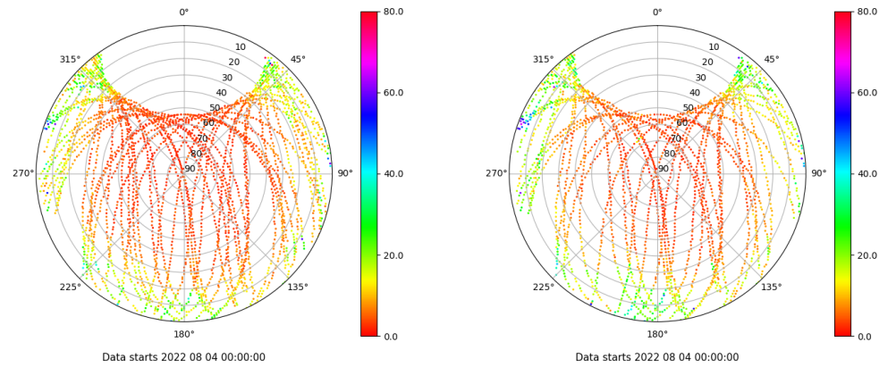
Skyplot for station IZAN. Parameter M1C Data file IZAN00ESP_R_2022216.xtr Skyplot for station IZAN. Parameter M2S Data file IZAN00ESP_R_2022216.xtr
