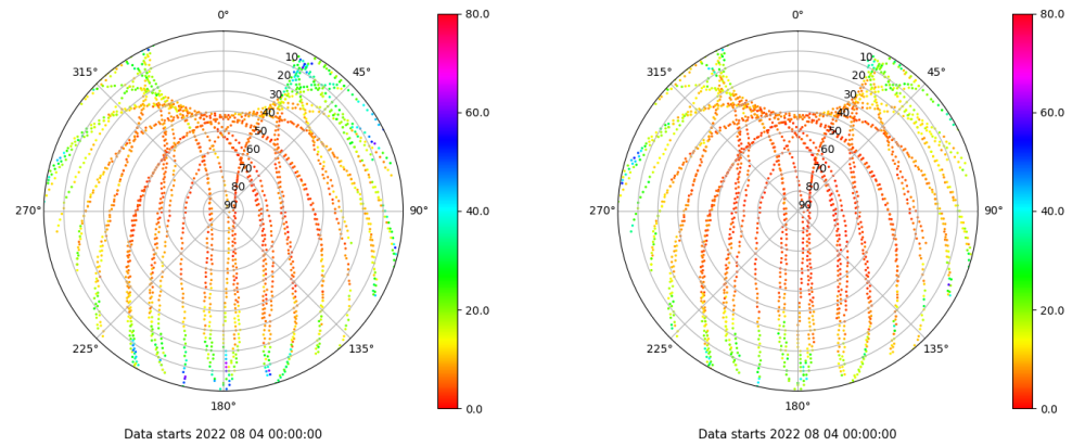
Skyplot for station IZAN. Parameter M1C Data file IZAN00ESP_R_2022216.xtr Skyplot for station IZAN. Parameter M2C Data file IZAN00ESP_R_2022216.xtr
